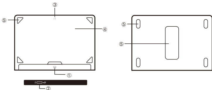
① Plateau soutenant ② Bouton d'ajustement ③ Ouverture ④ Panneau de support ⑤ Caoutchouc antidérapant
