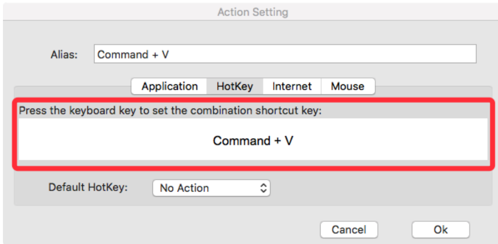
Afbeelding 3-28: Actie-instelling
