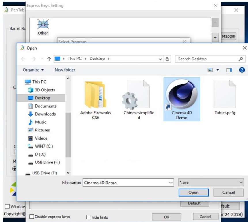
Afbeelding 3-13: Selecteer Programma
