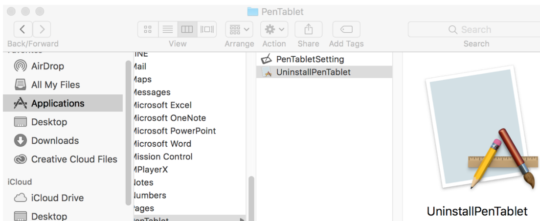
Afbeelding 4-1: Mac de-installeren
