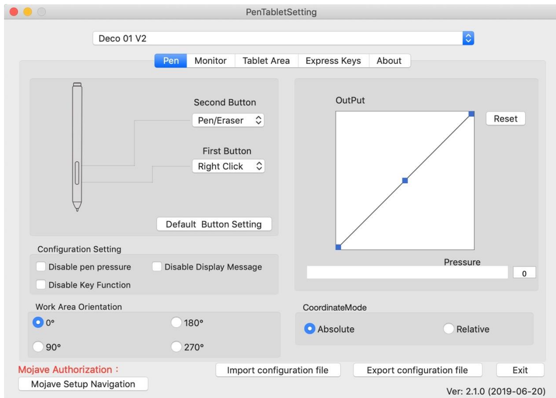
Afbeelding 3-16: Pen
