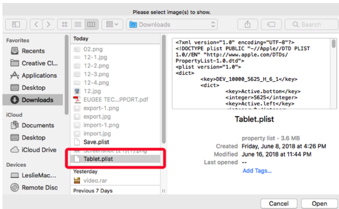
Afbeelding 3-23: Configuratiebestand importeren
