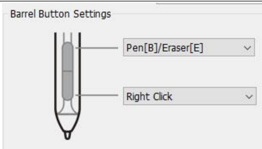
Afbeelding 3-2: Penfunctie-instellingen
