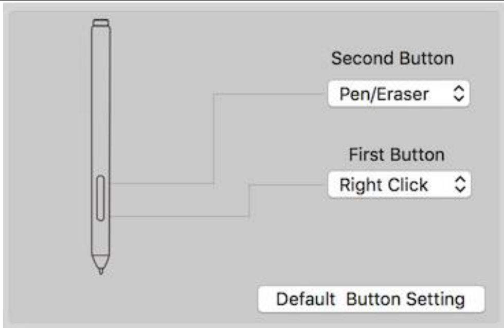
Afbeelding 3-17 Pen
