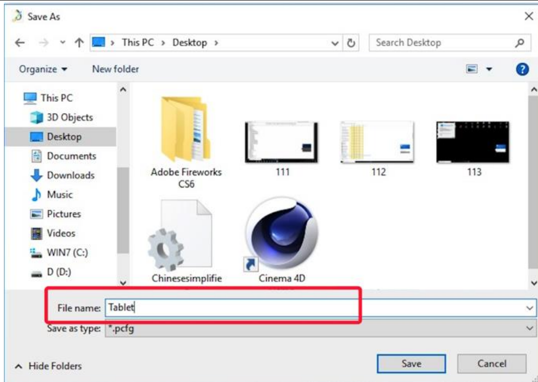
Afbeelding 3-6: Exportprofiel
