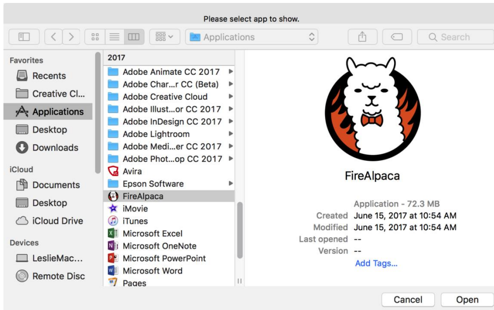
Afbeelding 3-30: Selecteer Programma
