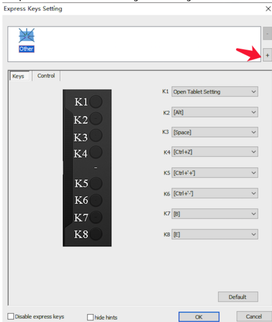
Afbeelding 3-12: Selecteer Programma
