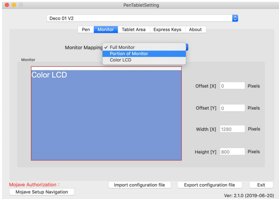
Afbeelding 3-25: Monitor
