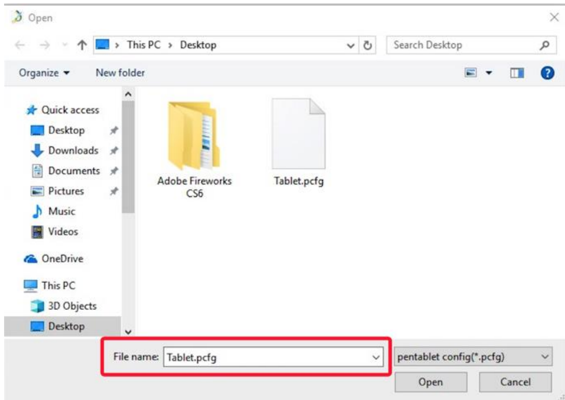
Afbeelding 3-7: Importprofiel
