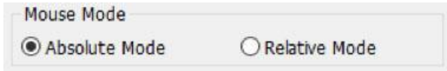
Afbeelding 3-4: Muismodus
