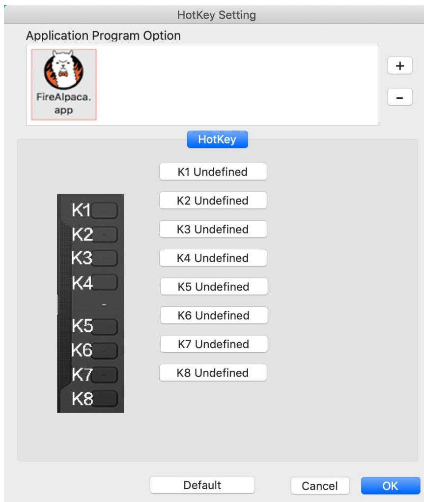
Afbeelding 3-31: Sneltoets
