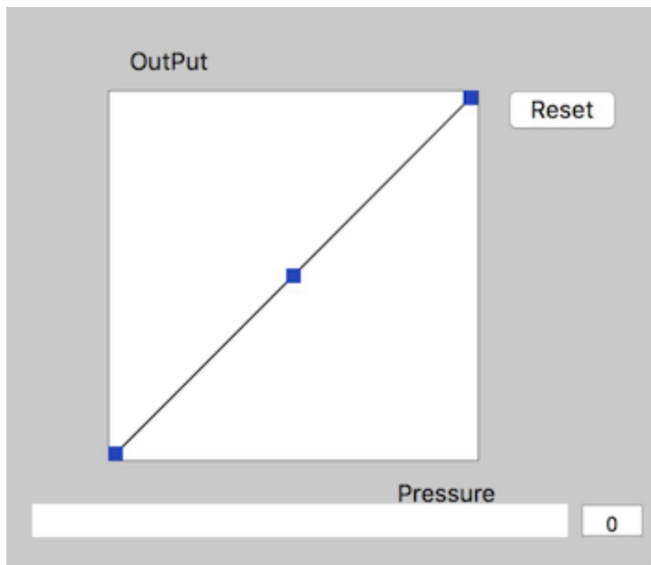
Afbeelding 3-20: Output
