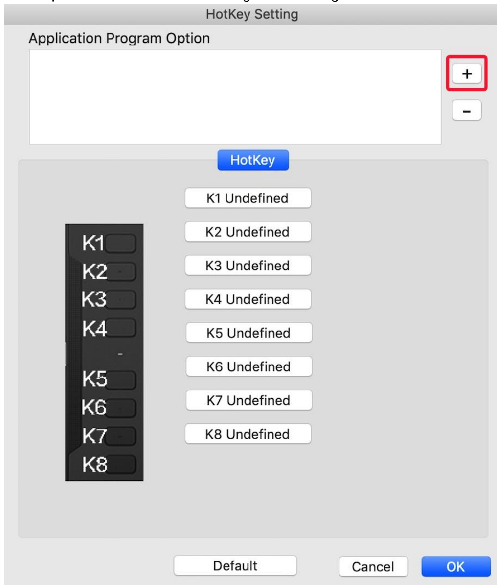
Afbeelding 3-29: Selecteer Programma
