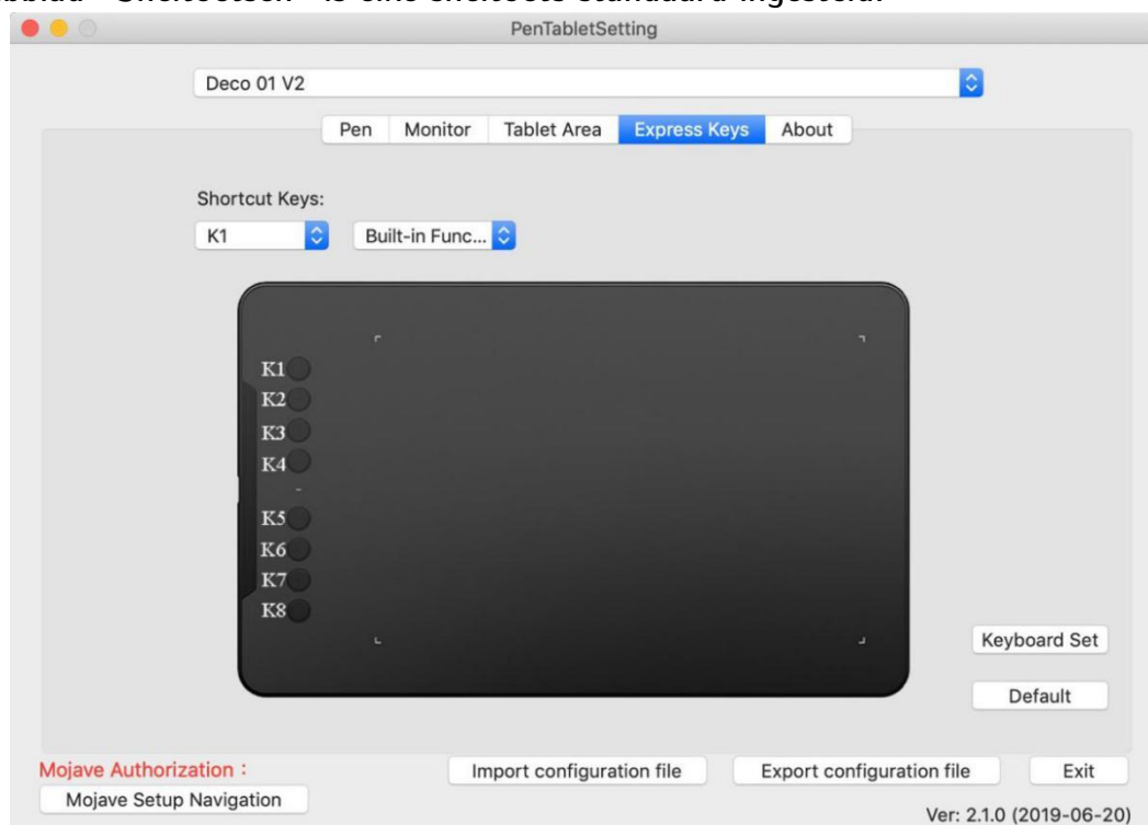
Afbeelding 3-27: Sneltoetsen
