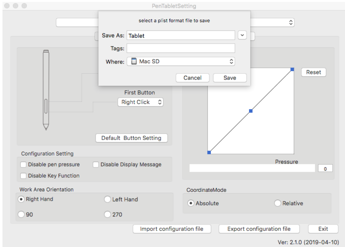
Afbeelding 3-22: Configuratiebestand exporteren
