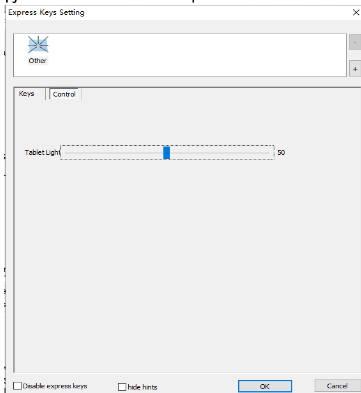
Afbeelding 3-14: Bediening
