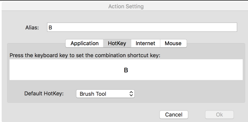
Afbeelding 3-32: Actie-instelling
