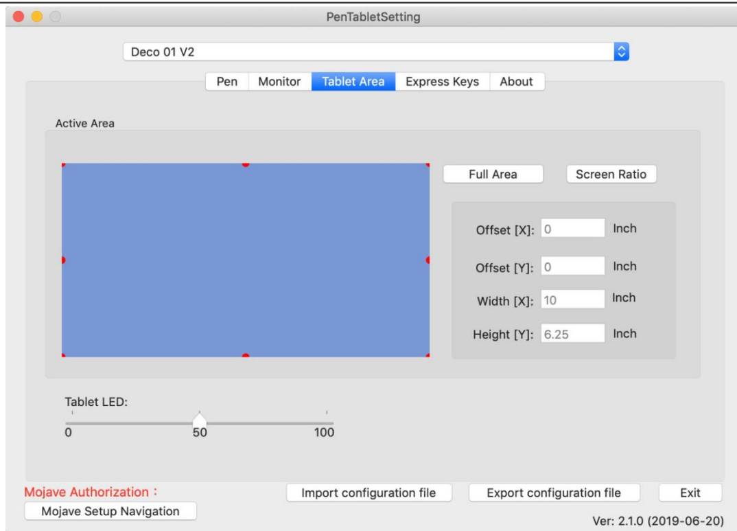
Afbeelding 3-26: Volledig bereik
