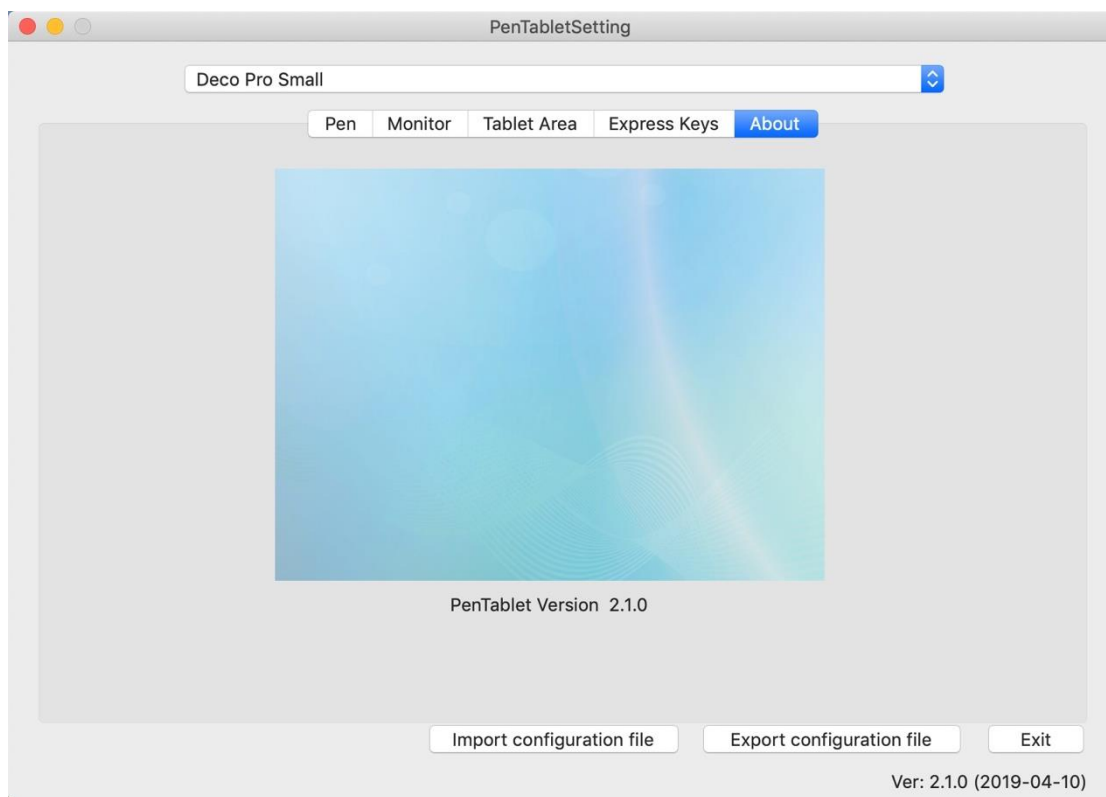
Afbeelding 3-33: Over
