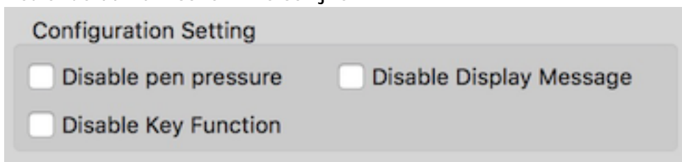
Afbeelding 3-18: Configuratie-instelling
