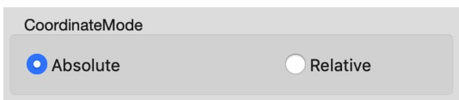
Afbeelding 3-21: Coördinatenmodus
