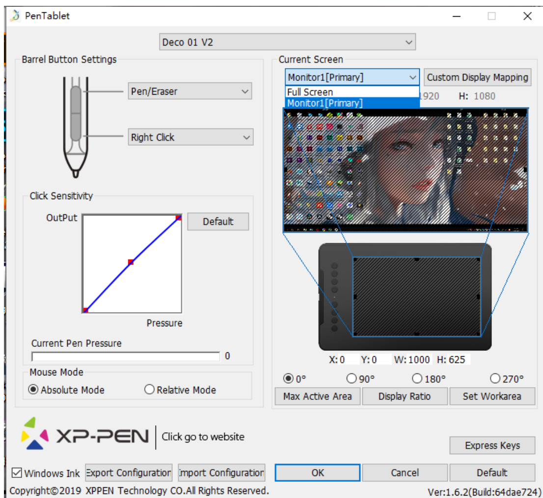
Afbeelding 3-1: Gebruikersinterface
