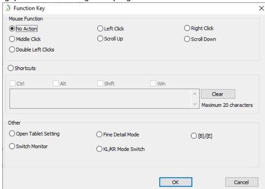
Afbeelding 3-11: Functietoets
