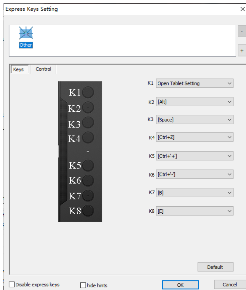
Afbeelding 3-10: Toetsen 10
